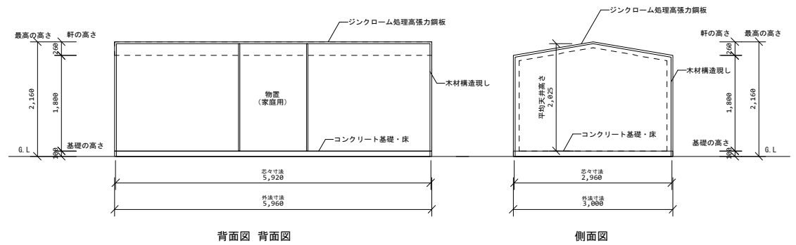
断面図 1/100
