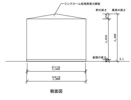
立面図 1/100
