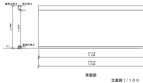
立面図 1/100
