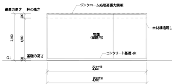
背面図
