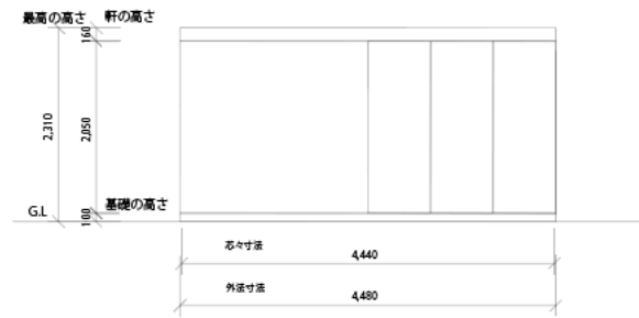
正面図
