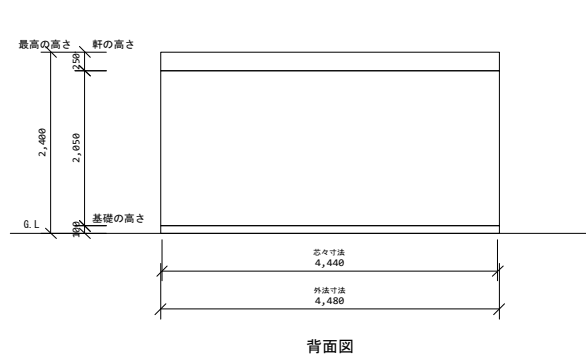
立面図 1/100
