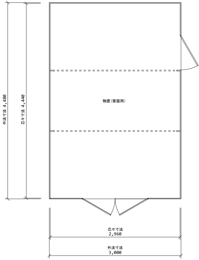
平面図 1/50
