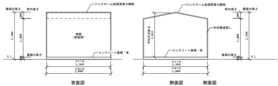
断面図 1/100
