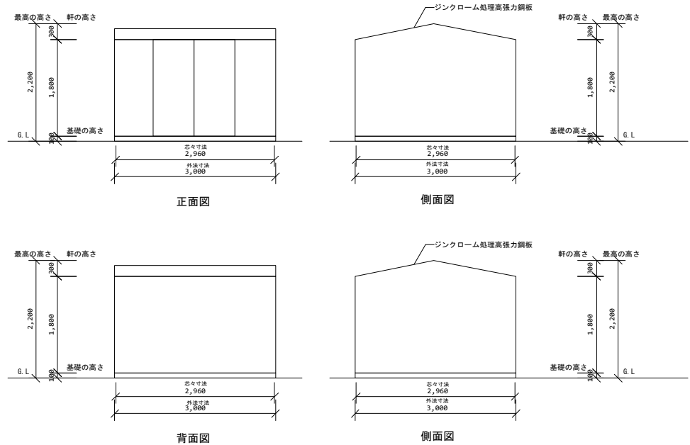
立面図 1/100
