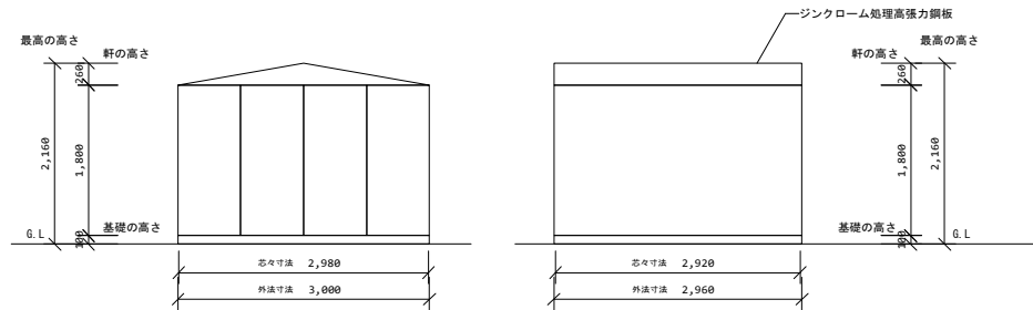
正面図
