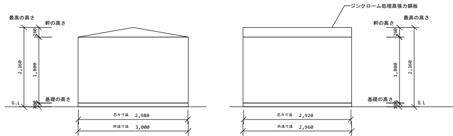
背面図
