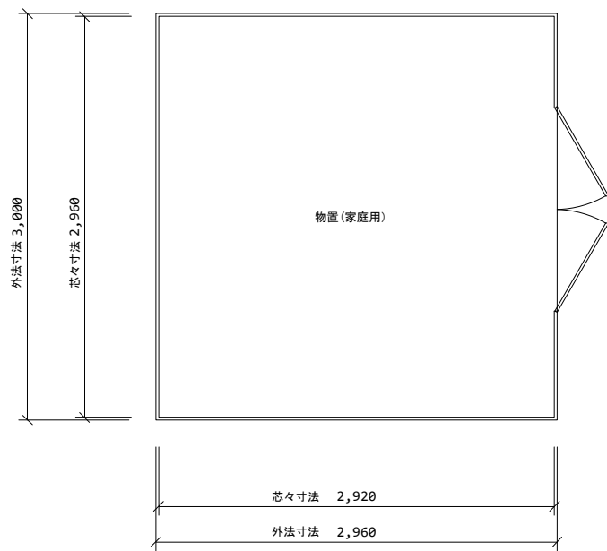
平面図 1/50
