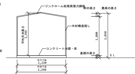
側面図
