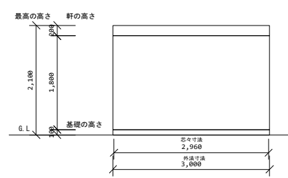
正面図
