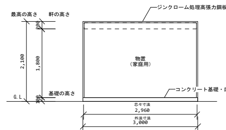
背面図
