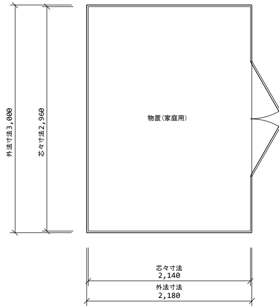
平面図 1/50
