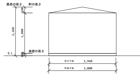
背面図
