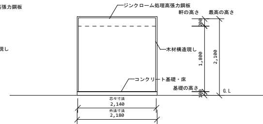
側面図
