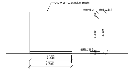
側面図(断面図)
