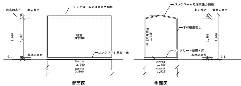
断面図 1/100
