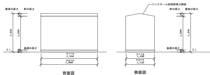
立面図 1/100
