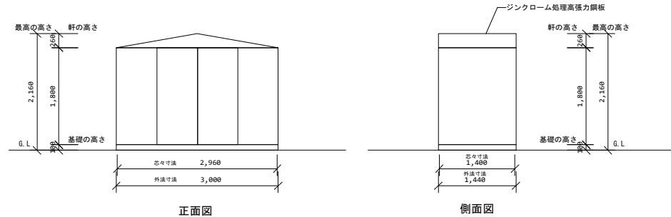
正面図
