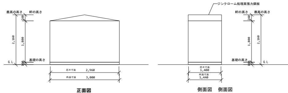
背面図
