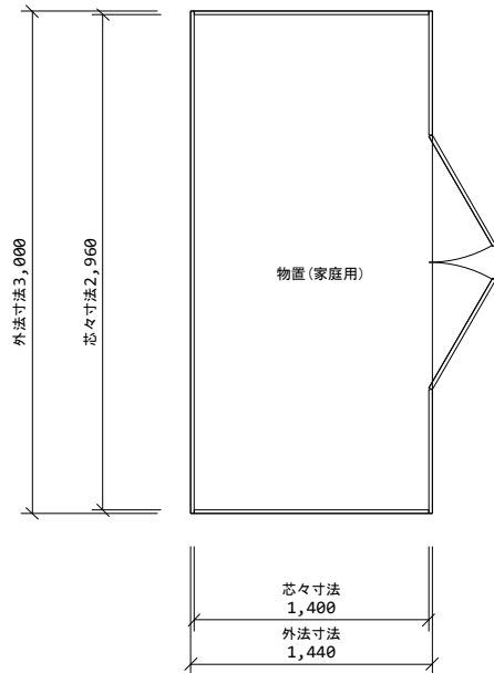
平面図 1/50
