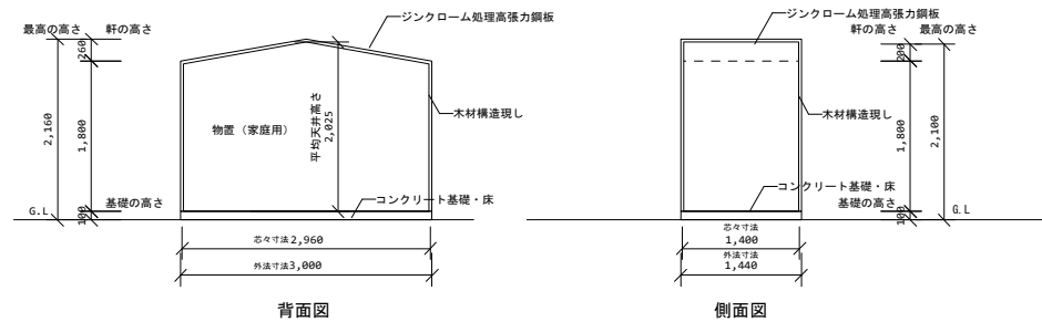
背面図
