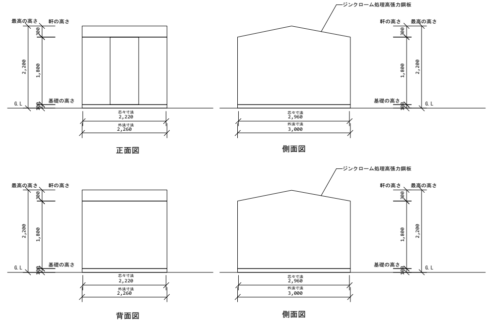
立面図 1/100
