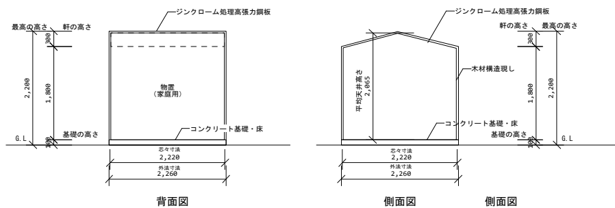
断面図 1/100
