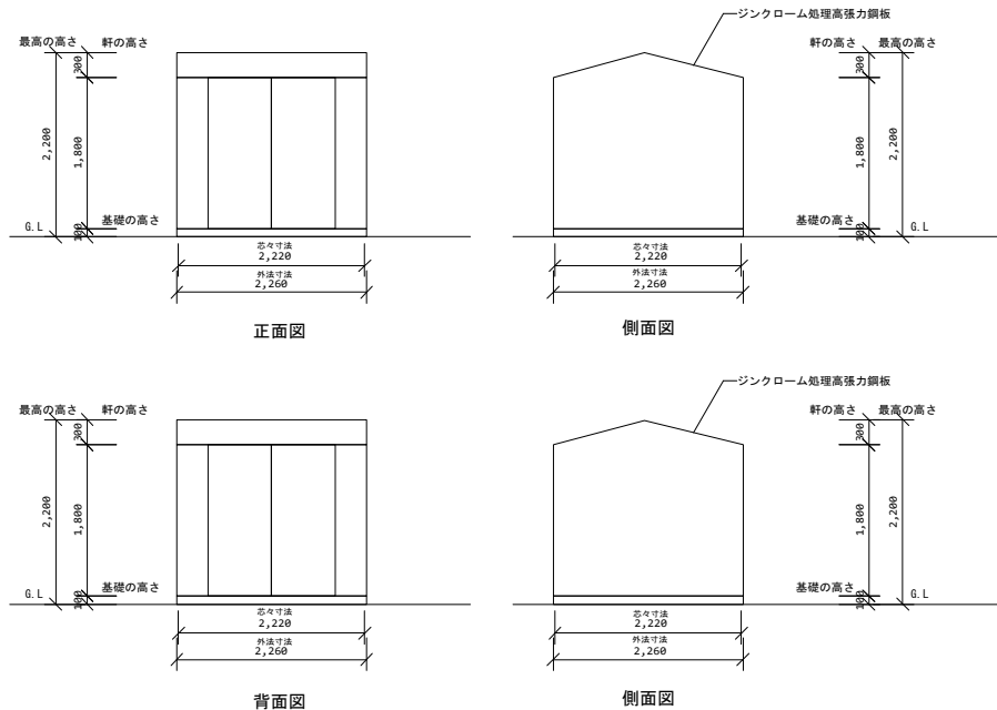
立面図 1/100
