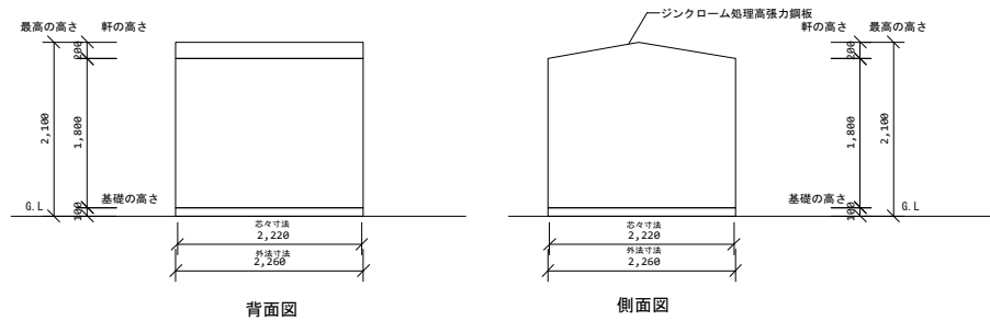
立面図 1/100
