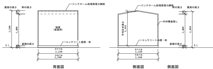
断面図 1/100
