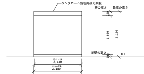
側面図
