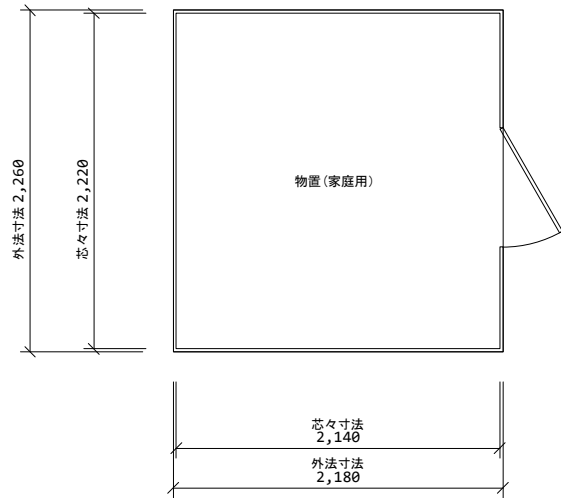
平面図 1/50
