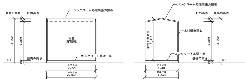
断面図 1/100
