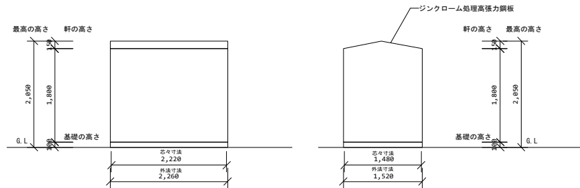
立面図 1/100
