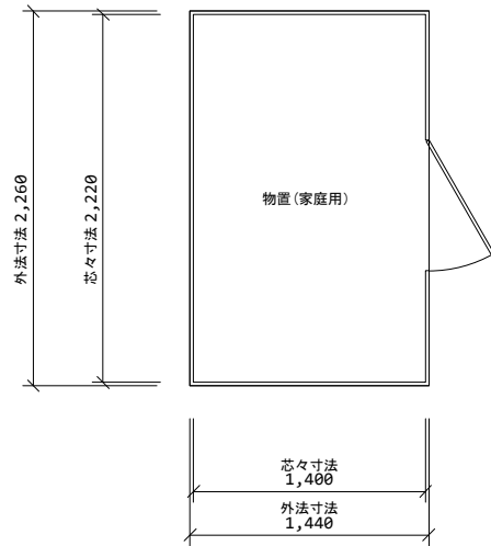
平面図 1/50
