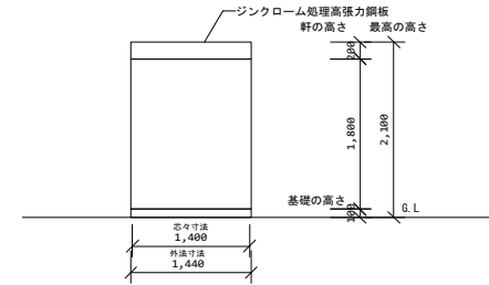
側面図
