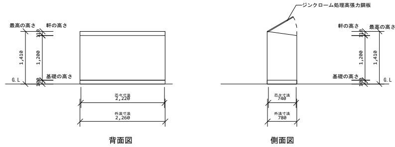
立面図 1/100
