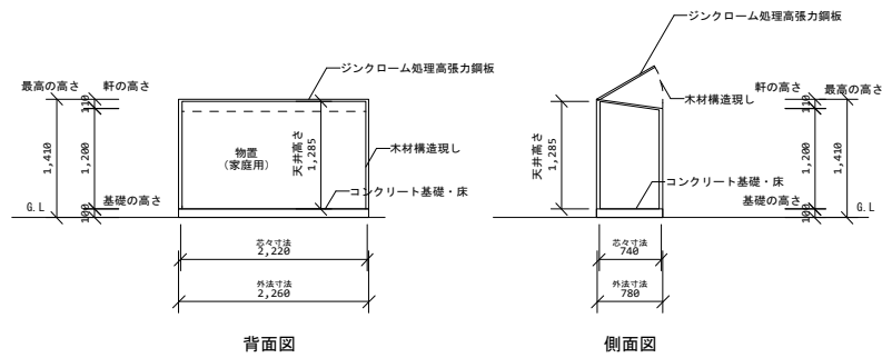
断面図 1/100
