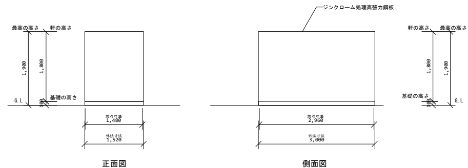
立面図 1/100
