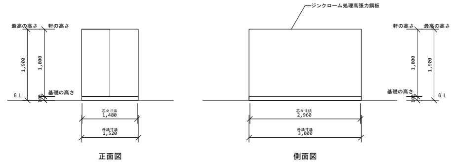
正面図
