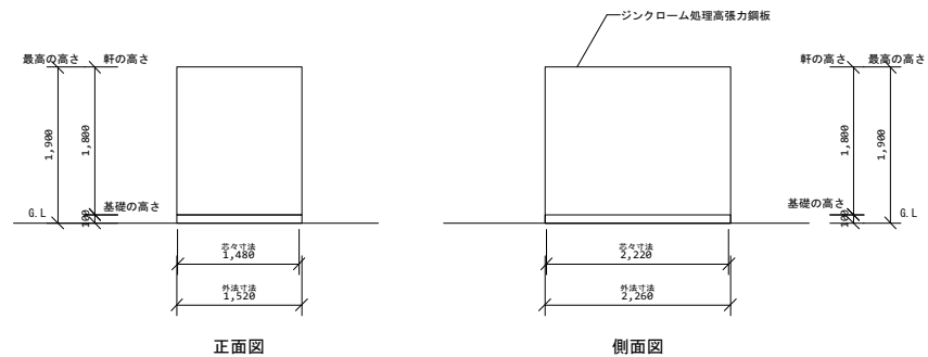
立面図 1/100
