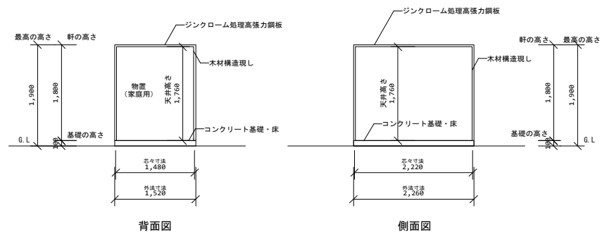
断面図 1/100
