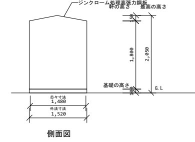
立面図 1/100
