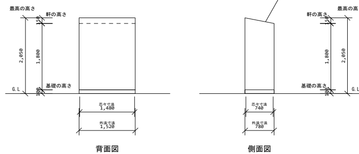
立面図 1/100
